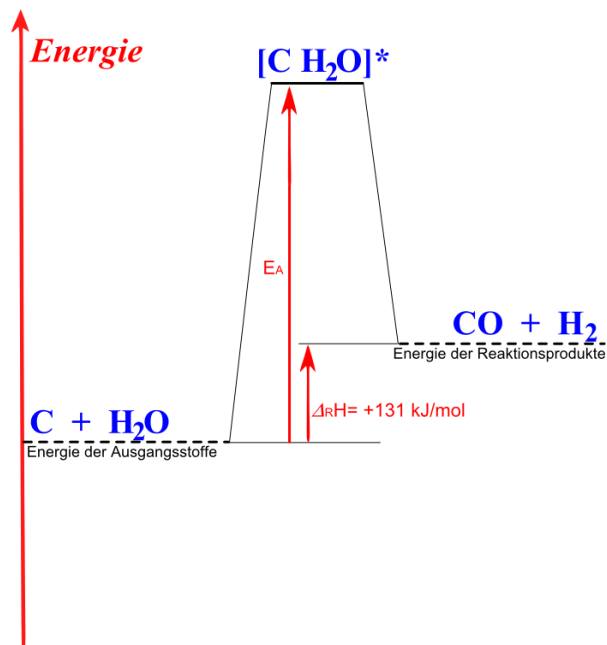
einfaches Energie-Niveau-Schema einer Reaktion mit (notwendiger) Energie-Aufnahme
