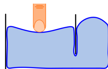
beeinflusstes Gleichgewicht
