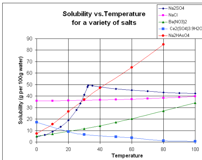
Löslichkeit ausgewählter Salz bei verschiedenen Temperaturen Q: de.wikipedia.org (Walkerma)
