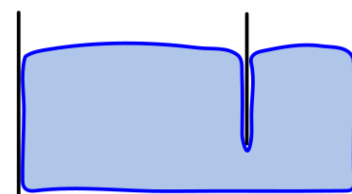
unbeeinflusstes Gleichgewicht
