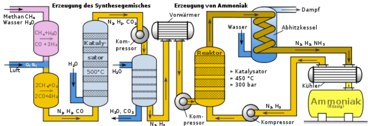
HABER-BOSCH-Verfahren Q: de.wikipedia.org (Sven)
