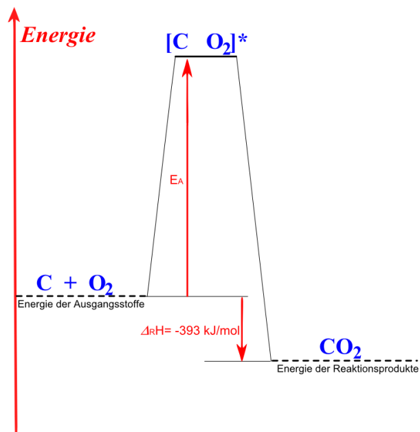
einfaches Energie-Niveau-Schema einer exothermen Reaktion
