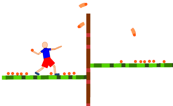
Modell einer einfachen Reaktion
