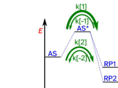
Beispiel für z.B. kinetisch bedingte Geschwindigkeits-Konstanten
