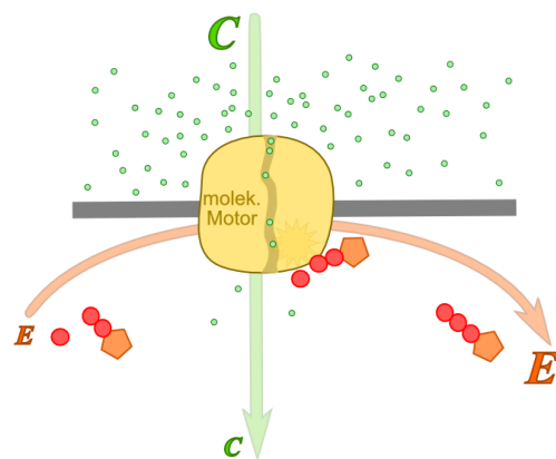
osmo-chemische Kopplung
