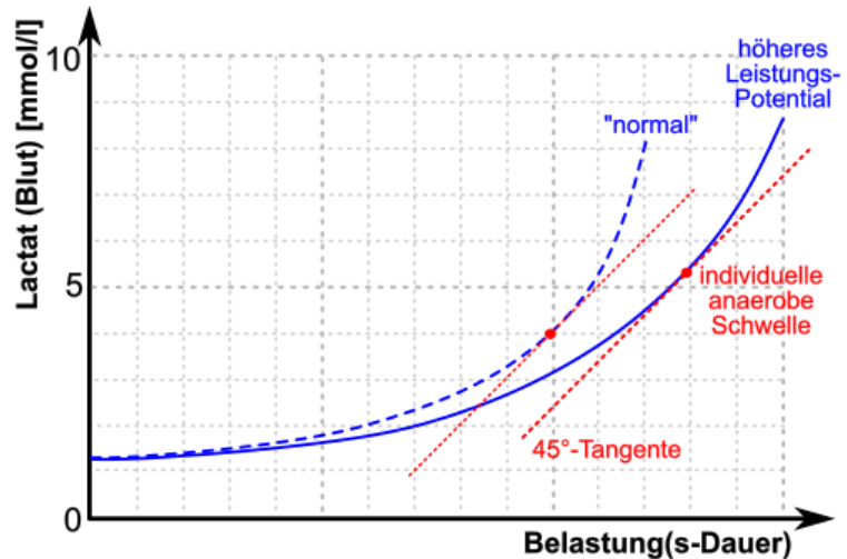
Abhängigkeit Blut-Lactat von der Belastung mit individueller anaerober Schwelle nach SIMON
