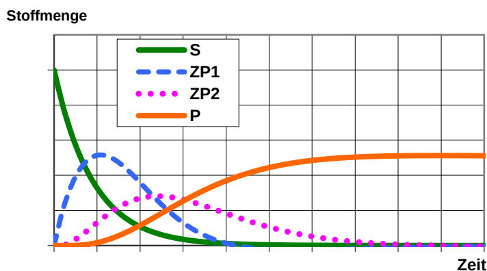
Stoff-Mengen / -Konzentrationen in einer (Modell-)Reaktions-Folge mit Rückkopplung (auf die 1. Reaktion)
