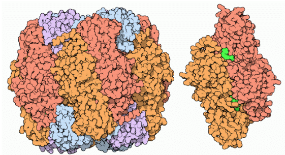
RUBISCO (rechts: einzelnes Dimer (1 von 8), wie es bei Bakterien vorkommt) Q: www.rcsb.org [Molecule of the Month]
