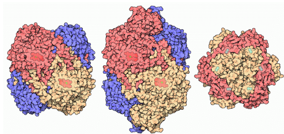
Katalasen verschiedener Organismen (Molekül-Modelle)
