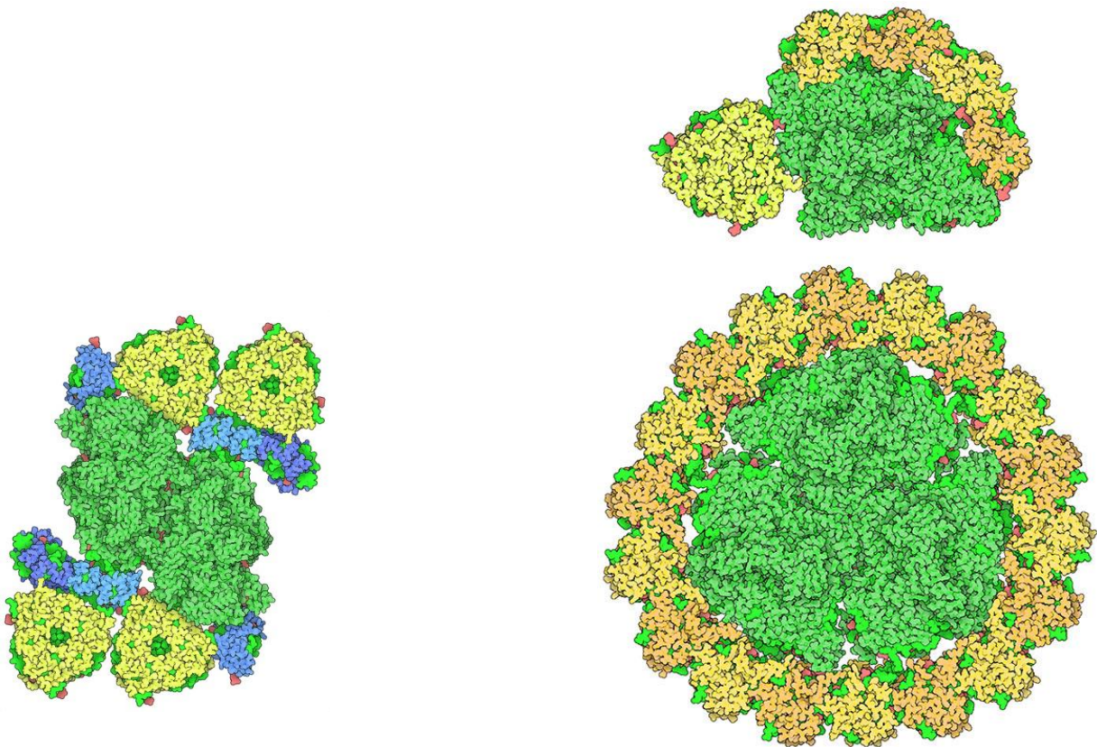
Photosysteme Dimer (links); Segment (oben) und vollständiger Super-Komplex (rechts unten) Q: rcsb.org [Molecule of the Month]
