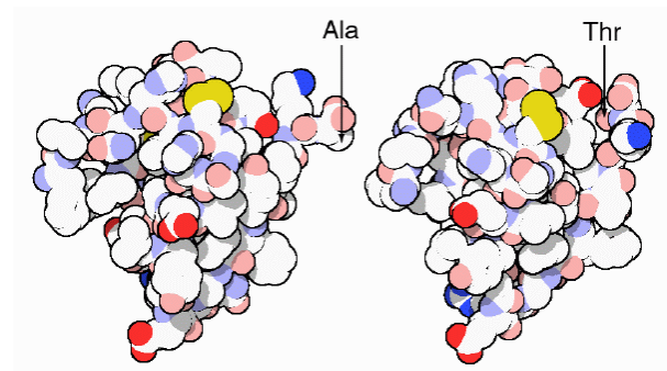
Insuline von Schwein und Mensch Q: rcsb.org [Molecule of the Month]
