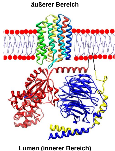
Rhodopsin in einer Membran; weiteres plasmatisches Protein Q: commons.wikimedia.org (Dpryan)
