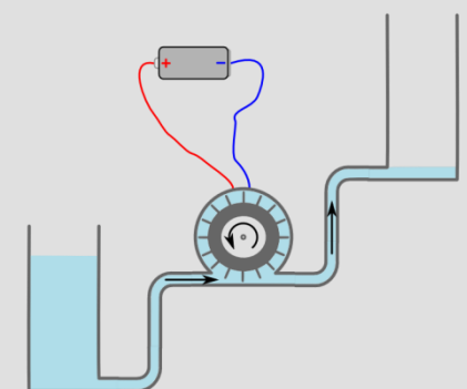
endergoner (erzwungener) Prozeß
