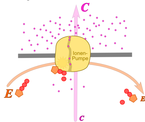
chemo-osmotische Kopplung (c .. Konzentration)
