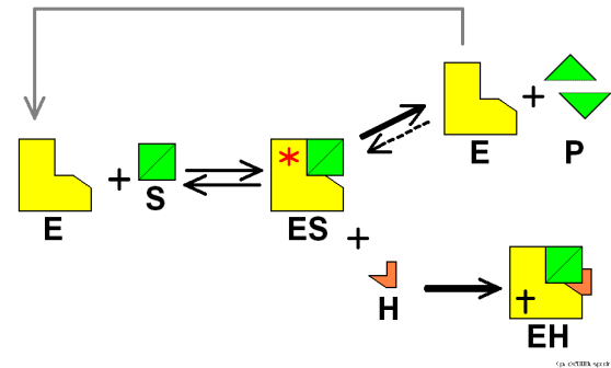
Ablaufschema einer irreversiblen unkompetitiven Hemmung
