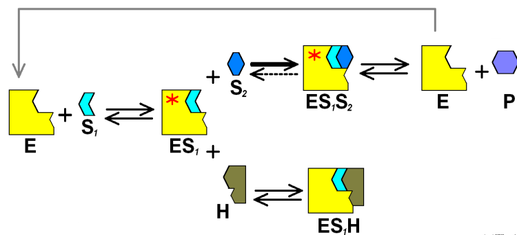
Ablaufschema eines Zwei-Substrat-System's mit Hemmung
