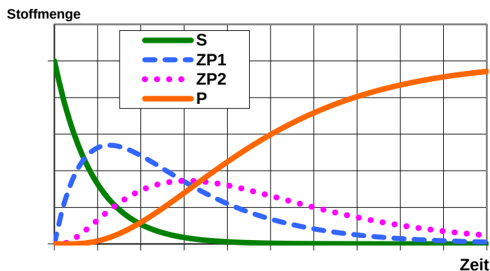
Stoff-Mengen / -Konzentrationen in einer (Modell-)Reaktions-Folge ohne Rückkopplung
