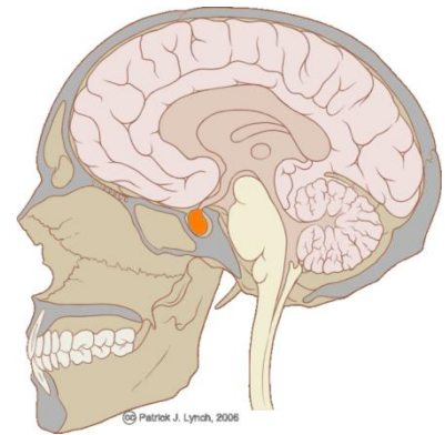
Lage der Hypophyse (orange) Q: de.wikipedia.org (Patrick L. Lynch)
