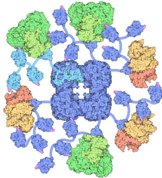
Pyruvatdehydrogenase-Enzym-Komplex (Molekül-Modell, schematisch) Q: rcsb.org [Molecule of the Month]
