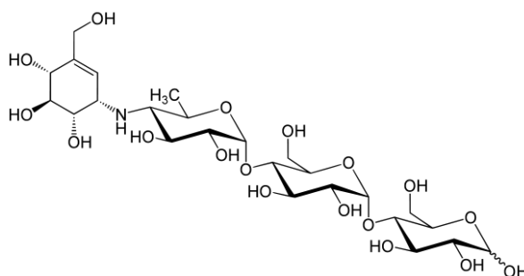
Acarbose (Strukturformel) Q: de.wikipedia.org (Yikrazuul)
