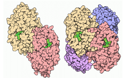
Enzym (Alkoholdehydrogenase), Dimer und Tetramer
