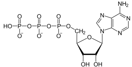
Triphosphat Ribose Adenin ATP-Molekül; Strukturformel Q: de.wikipedia.org (NEUROtiker)
