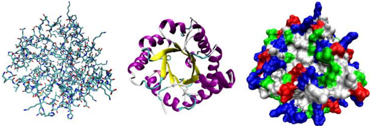
Triose-Phosphat-Isomerase (Atom-Stab-, Band- u. Raum-Modell) Q: en.wikipedia.org
