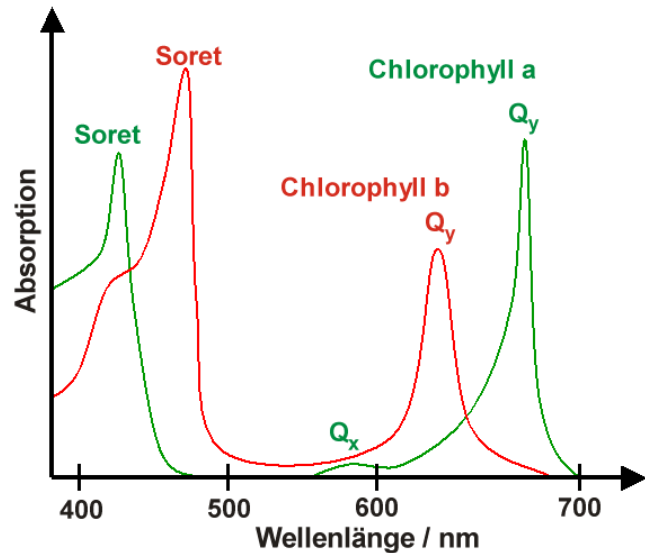
Absorptions-Spektren verschiedener Chlorophylle
