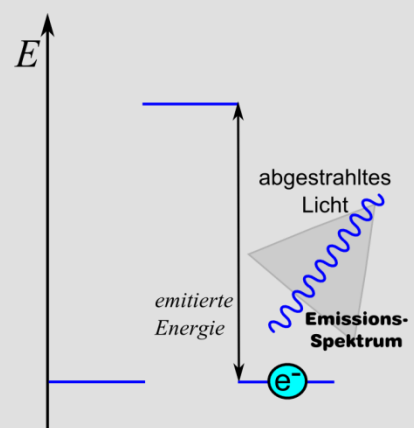
Emmission (hier blaues Licht)
