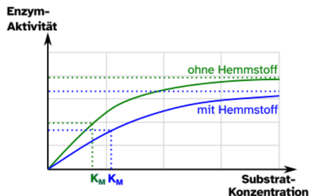
Substrat-Abhängigkeit bei konstanter Hemmstoff-Konzentration
