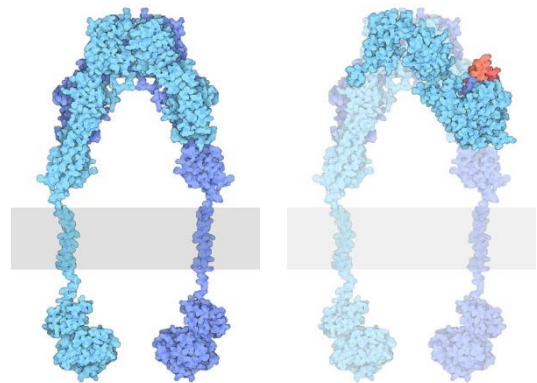
Insulin-Rezeptor ohne und mit Insulin Q: rcsb.org [Molecule of the Month]
