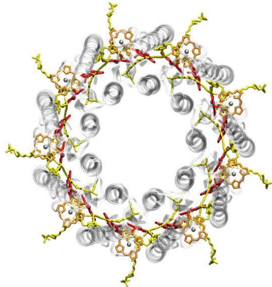
Chlorophyll-Komplex (Purpur-Bakterien)
