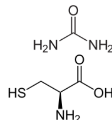
Harnstoff und Cystein Q: de.wikipedia.org (NEUROtiker)
