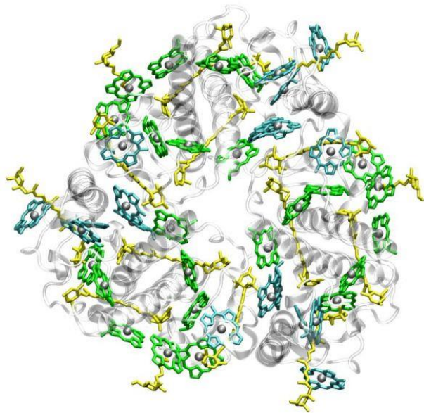
Chlorophyll-Komplex (LH2)
