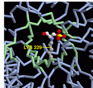
Aldolase-Tetramer und Ansicht eines aktiven Zentrums
