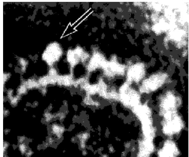
ATP-Synthase an der inneren Mitochondrien-Membran (EM-Aufnahme)
