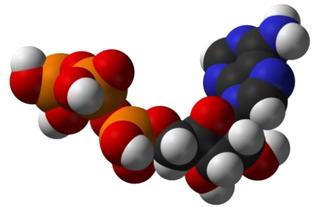
ATP-Molekül; Kalotten-Modell Q: de.wikipedia.org (Benjah-bmm27)
