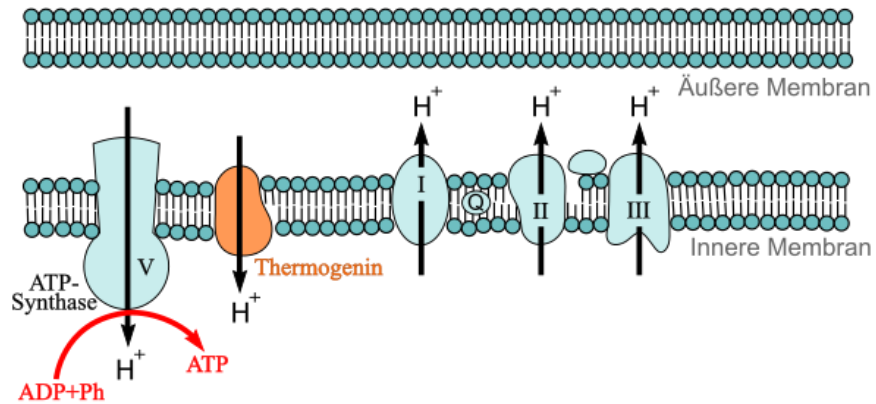
Thermogenin als Protonen-Kurzschluss
