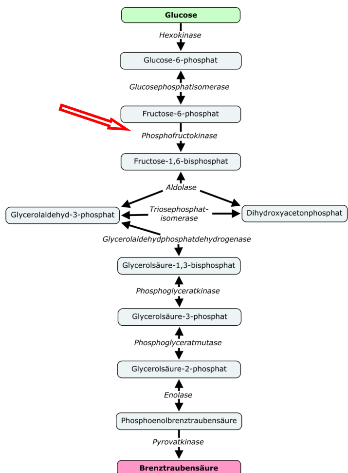
Überblick über den Metabolismus der Glycolyse
