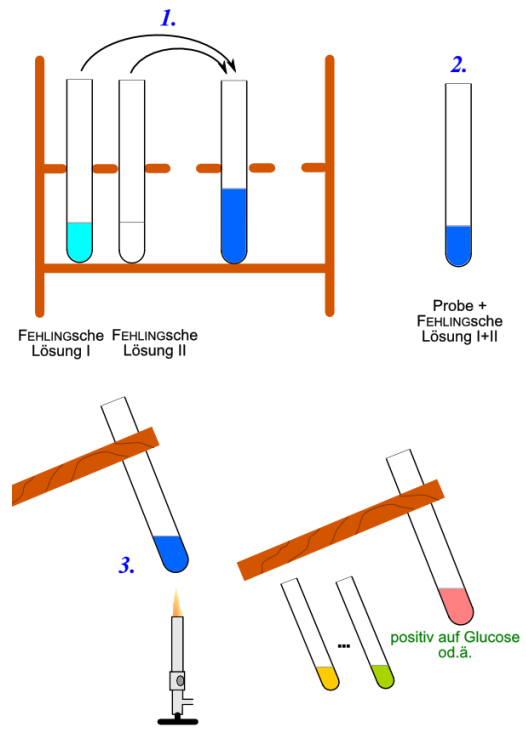
Glucose-Test nach FEHLING
