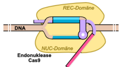
Cas-Komplex schematisch
