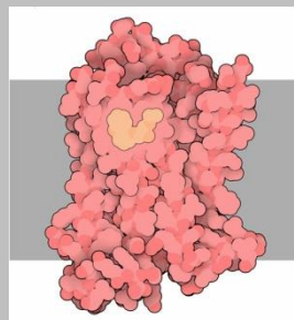
Modell eines Rezeptor (für Adrenalin); dieser besteht nur aus einem Monomer (Quartär-Struktur also gleich Tertiär-Struktur) Q: www.rcsb.org
