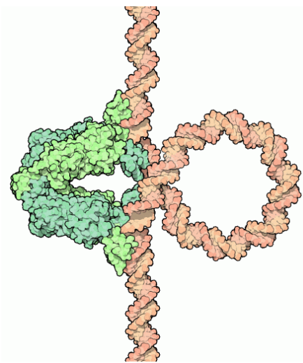
durch Laktat-Repressor gebildete DNA-Schleife Q: rcsb.org [Molecule of the Month]
