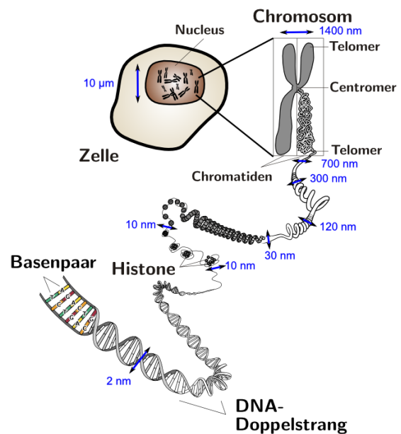
Gesamt-Übersicht zum Bau eines Chromosoms Q: de.wikipedia.org (Phrood (US-NioH); erweitert: lsp: dre)
