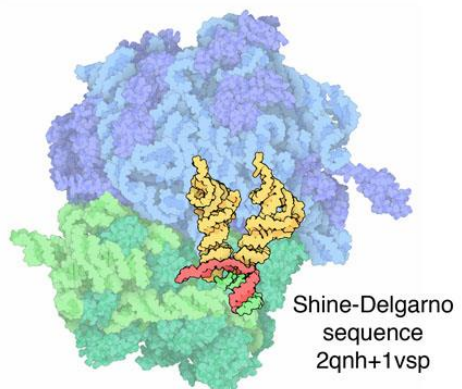
Start der Translation (mRNA (rot), tRNA (gelb)) Q: www.rcsb.org
