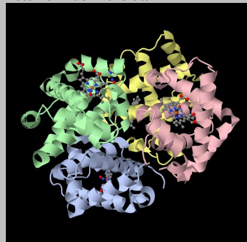
Band-Modell des Hämoglobin-Moleküls (Quartär-Struktur) die einzelnen Tertiär-Strukturen sind in verschiedenen Farben dargestellt Q: www.rcsb.org
