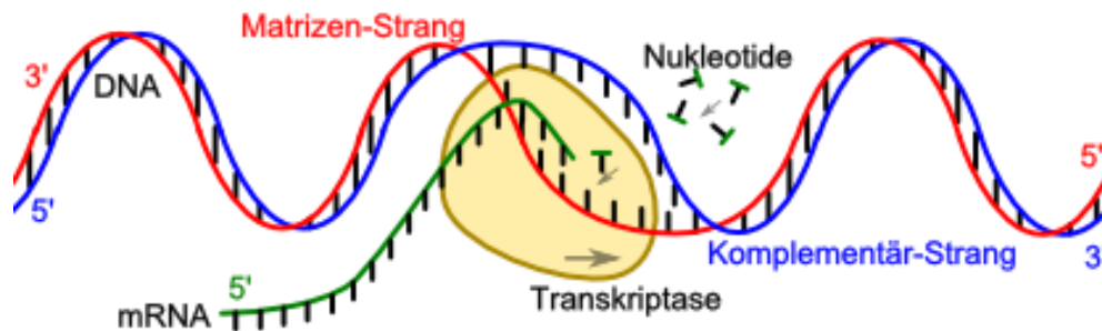
Transkription
