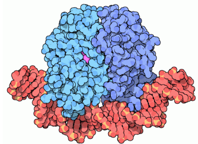
Repressor (blau) blockiert Operon (DNA-Molekül (rot)) Q: da.wikipedia.org (Giac83)
