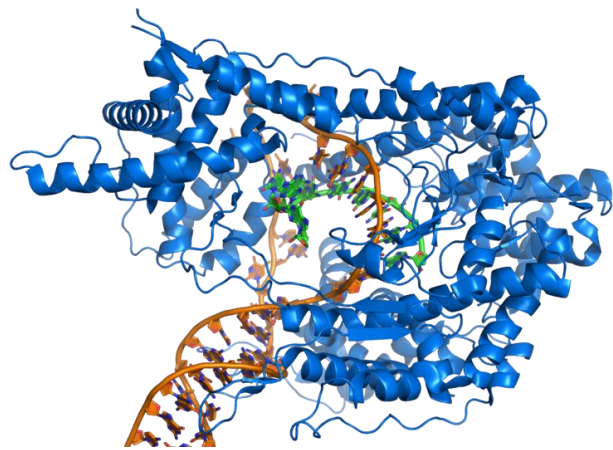
RNA-Polymerase (blau, Bänder-Modell) mit geweiteter DNA (orange-braun) und gebildeter mRNA (grün) Q: da.wikipedia.org (Thomas Spletstoeser)
