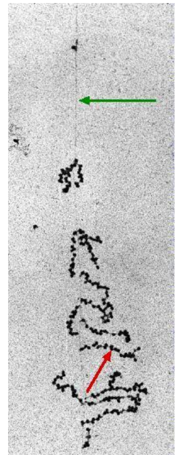
Polysom EM-Aufnahme
