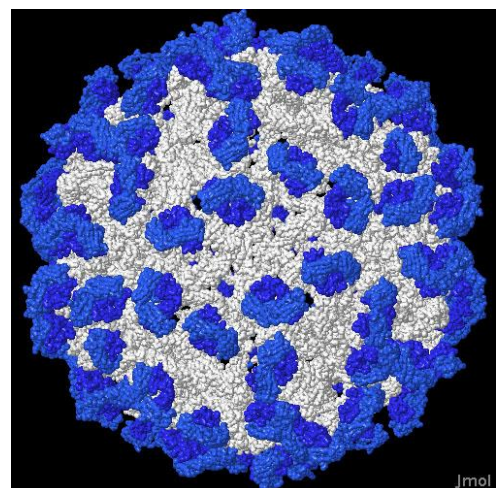
Dengue-Virus
