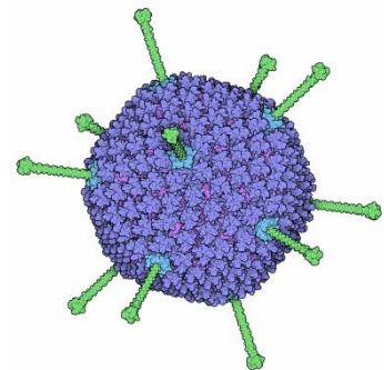
Adeno-Virus
