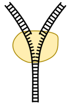
Y-Modell der Replikation
