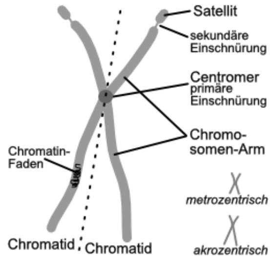
Metaphasen-Chromosom (Bau)
