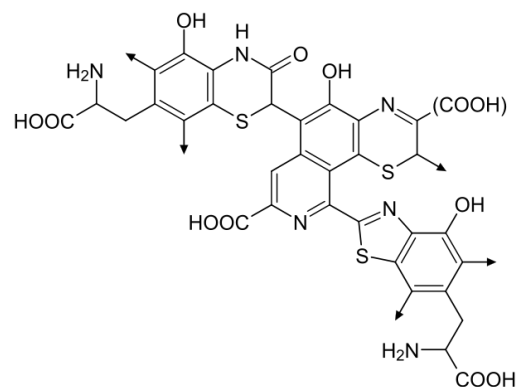
Phäomelanin
