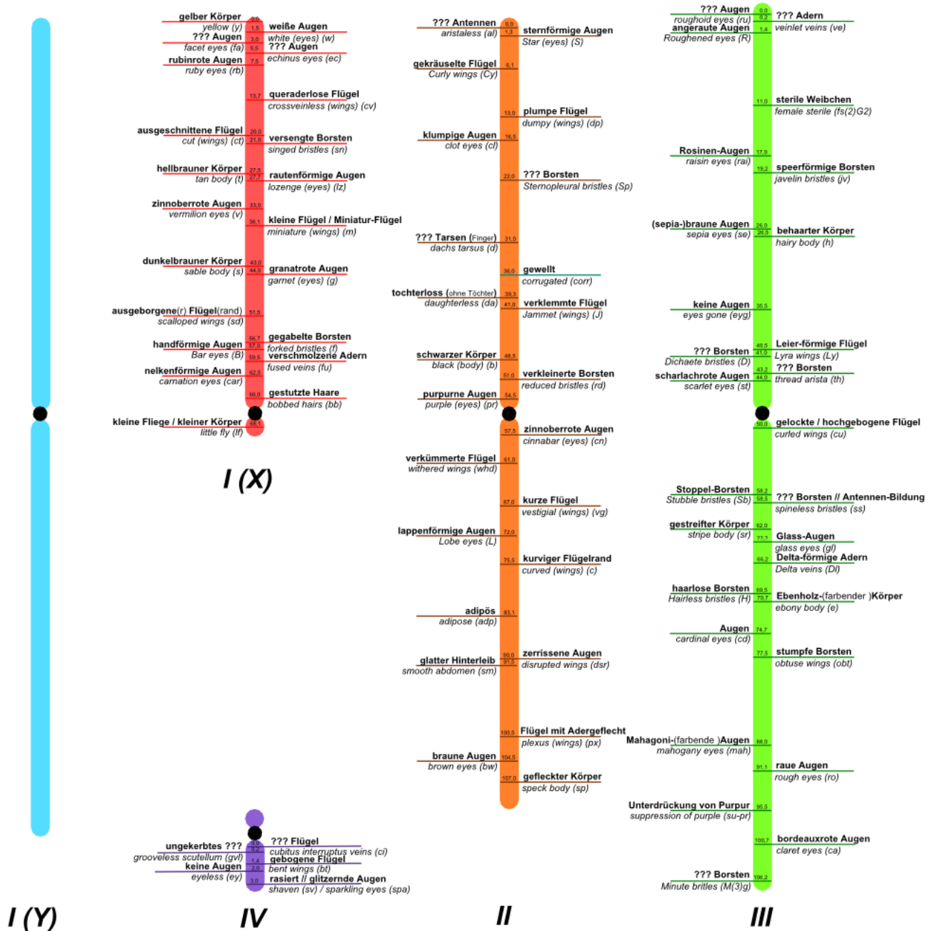
Chromosomen-Karte mit der Lage wichtiger / ausgewählter Gene für (s) Drosophila melanogaster klassische Chromosomen-Karte nach MORGAN
