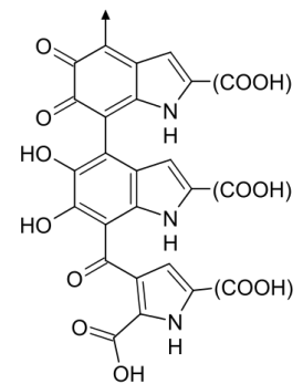
(Eu-)Melanin
